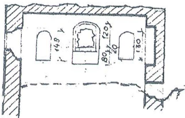
PJŪVIS 1-1
